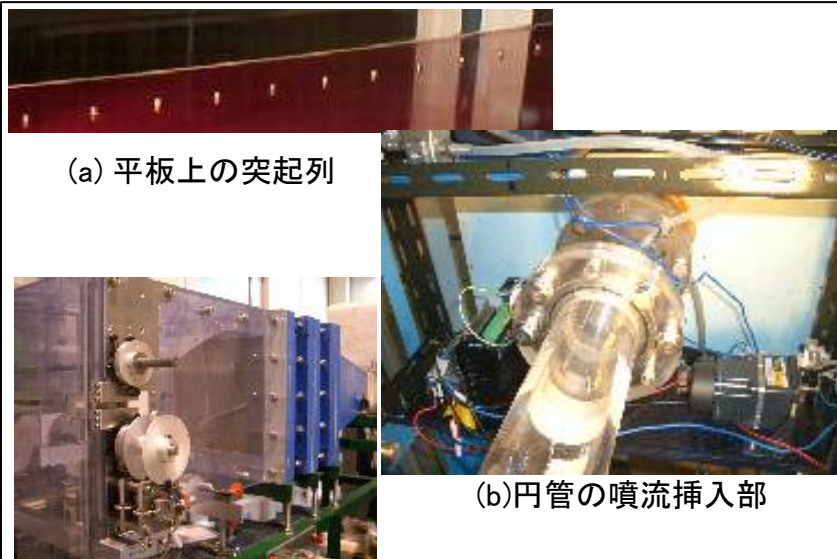
図1 本研究で使用する風洞
