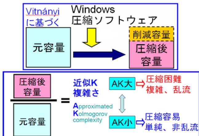
図2 コルモゴロフ複雑度解析の模式図
