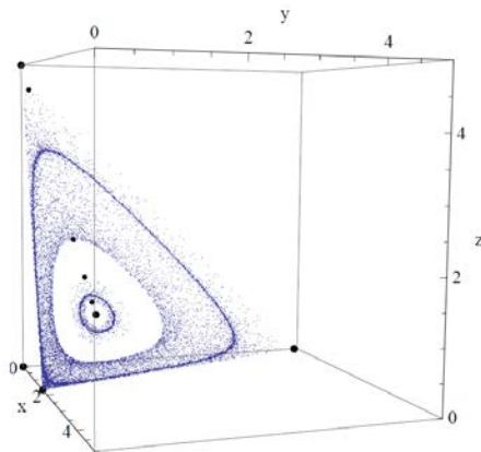
図1 解軌道: Zeemanの第27類での構成例
