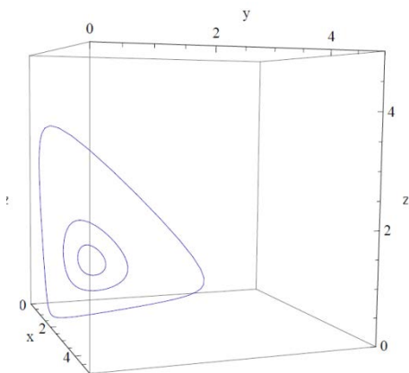
図2 極限周期軌道: Zeemanの第27類での構成例
