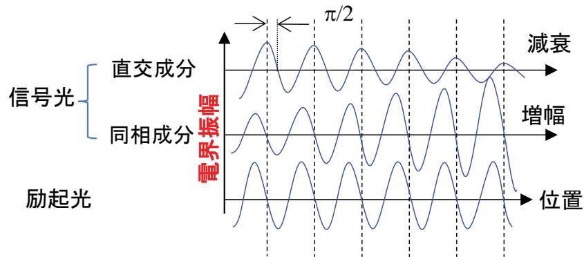
(a) PSAの基本動作
