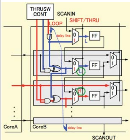
図2 TDC組込み型 バウンダリスキャン(TDCBS)
