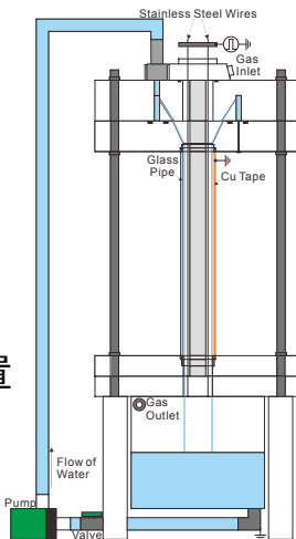
図4 ストリーマ放電
