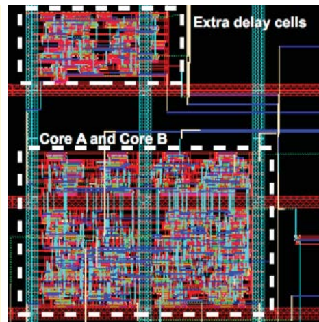
図3 TDCBSの試作 レイアウト図
