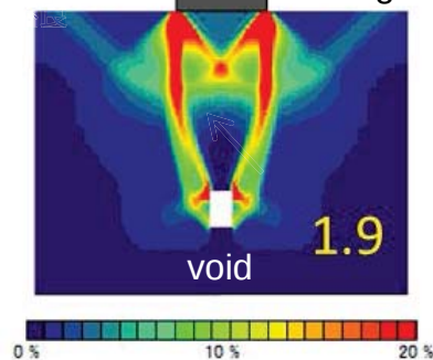
図2 空洞を有する地盤の支持力FEM解析
