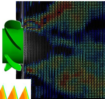
Fig.4 PIV result
