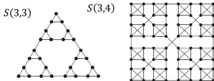
Fig.1 : Sierpiński graphs.
