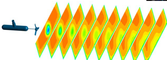
図5 プロペラタービンからの後流
