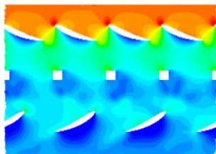
図3 翼列間流れ
