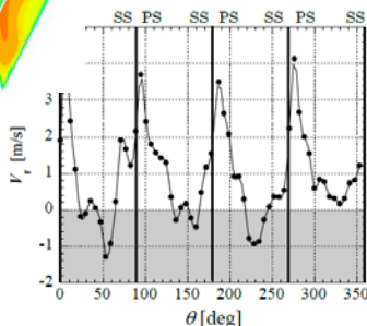
図8 ポンプ 出口速度分布
