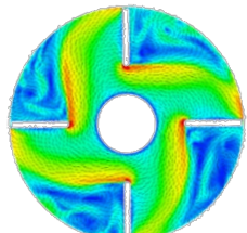
図7 ポンプ内の内部流れ
