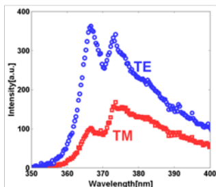
図4 UV-LEDからのELスペクトル
