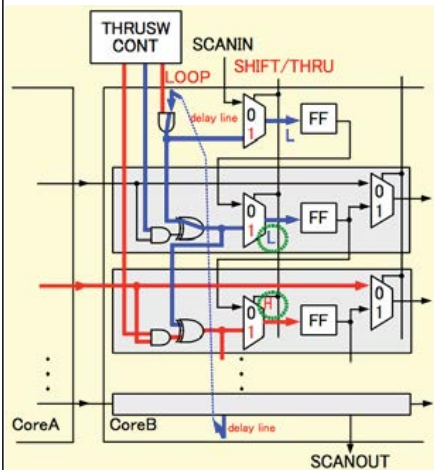
図2 TDC組込み型 バウンダリスキャン(TDCBS)
