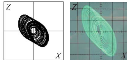
図2 カオスアトラクタ
