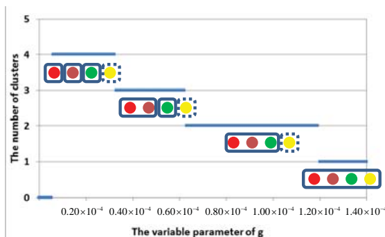
図5 結合強度によるクラスタ数の変化
