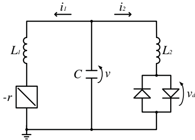
図1 カオス回路
