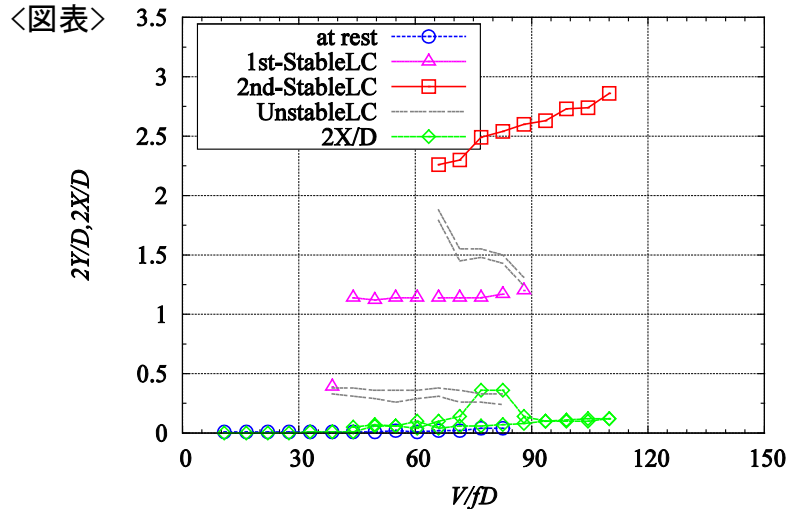
図1 直列2円柱の後流側円柱の主流直交方向と主流方向の振動応答の例(円柱間中心距離 L と直径 D の比 L/D=3 , スクルートン数 Sc=16.4 )
