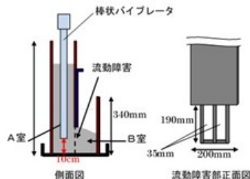
図-1 加振ボックス充填試験
