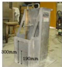
図-1 加振ボックス充填試験
