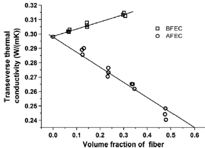
Fig. 2 Thermal conductivity vs. fiber content. DOI: 10.1016/j.compositesa.2012.02.020
