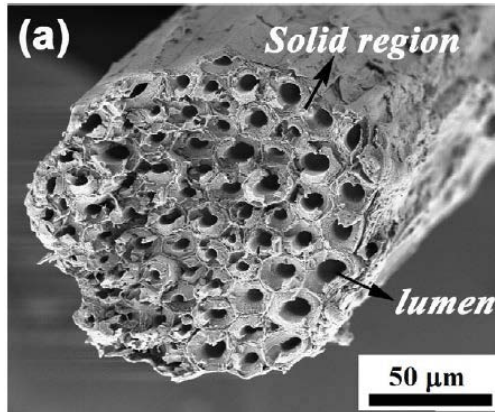
Fig. 1 Internal microstructure of natural fiber. DOI: 10.1016/j.matdes.2011.04.006
